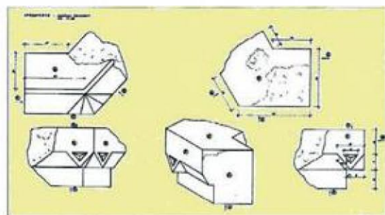
Crtež – detalj klesanih fragmenata
