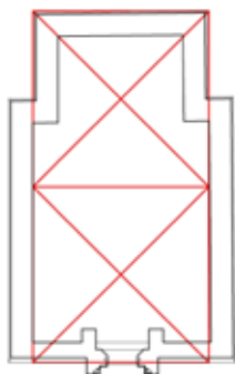
Oriovčić, crkva sv. Benedikta, 2. pol. 13. st. – kvadrangulacija tlocrta crkve. Crtao: Vedran Leš, analiza: Ratko Ivanušec
