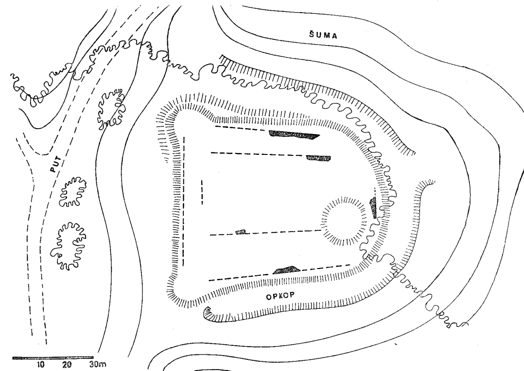
7 Mali (Gornji) Gradac, skica tlocrta prema sačuvanim ostacima, snimio i izradio inž. arh. Z. Horvat
