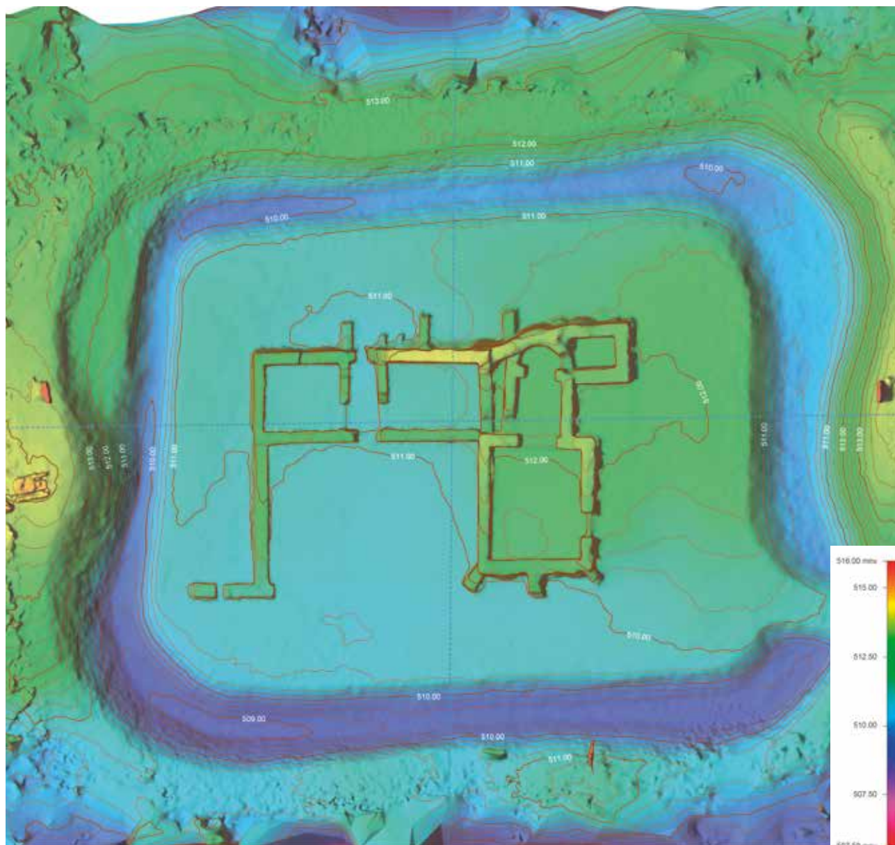
42 Model terena pavlinskog samostana sv. Petra i njegovih kasnijih pregradnji nakon dovršetka radova (izrada: „Vektra d.o.o.“, 2016.)
