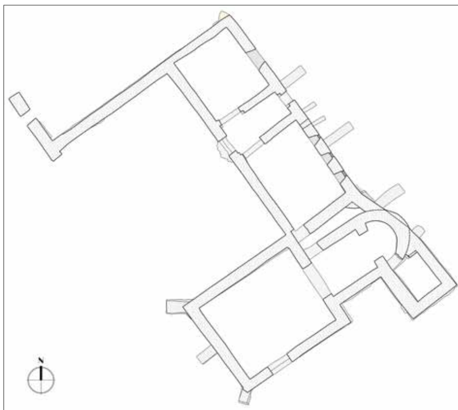
43 Tlocrt pavlinskog samostana sv. Petra i njegovih kasnijih pregradnji nakon dovršetka radova (izrada: „Vektra d.o.o.“, 2016.)
