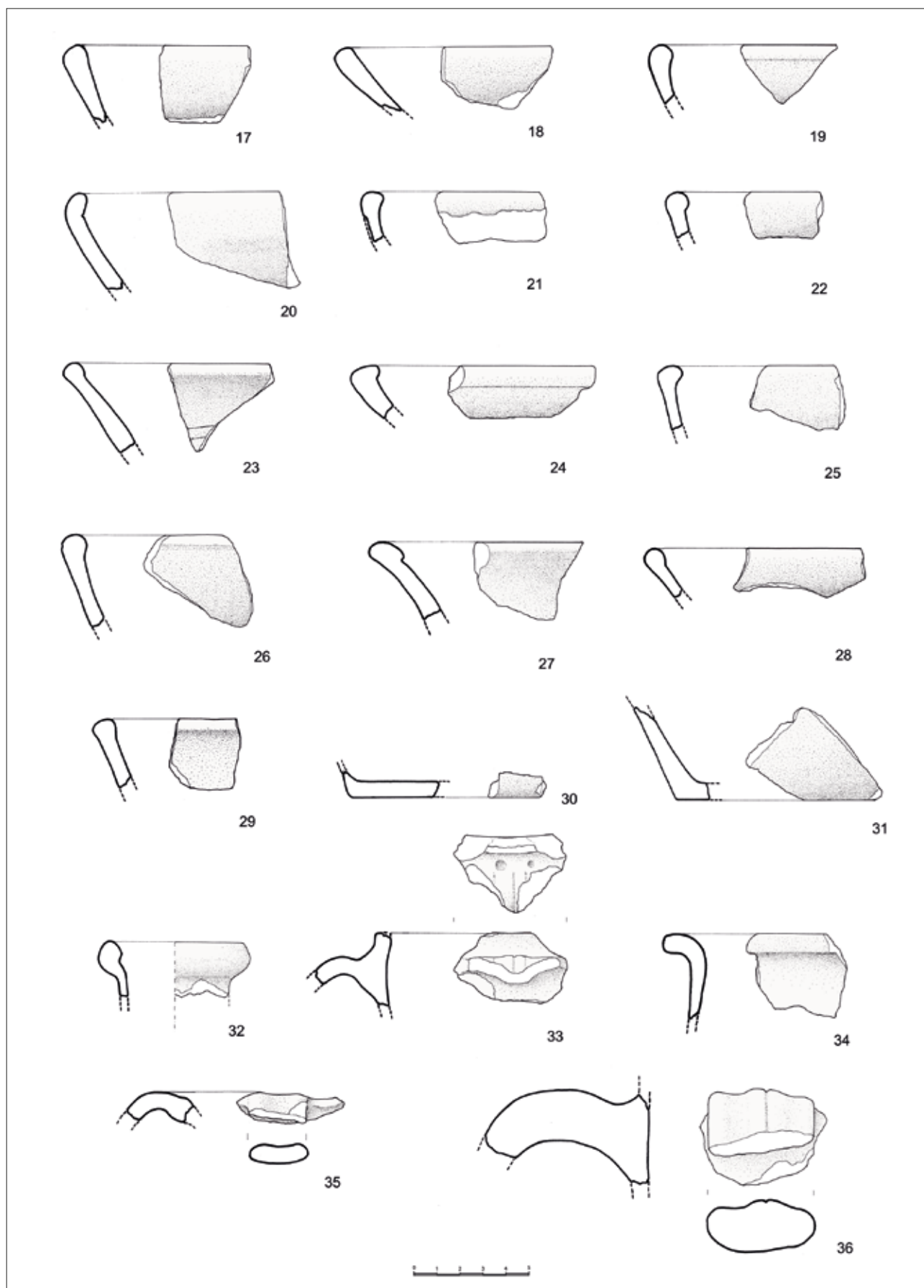
10 Rimski keramički nalazi pronađeni na Malom Petrovcu (crtež: M. Krmpotić, 2008.)
